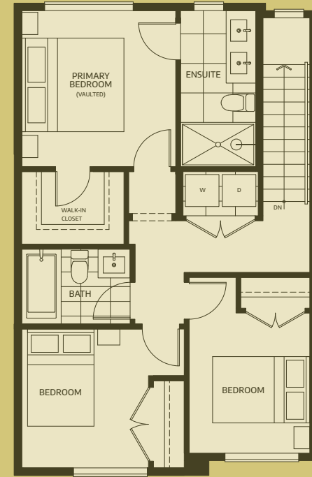
UPPER 642 SQFT
